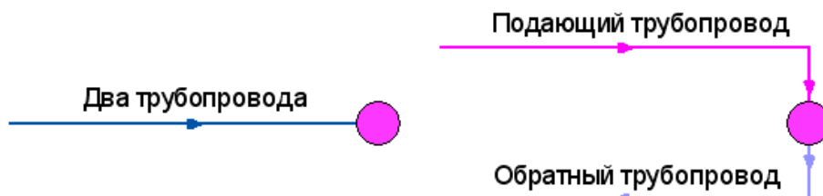
Рис. 3.12. Внешнее (слева) и внутреннее (справа) присоединение потребителя к тепловой сети
